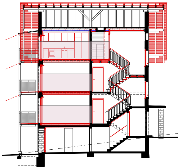
Schnitt C-C
