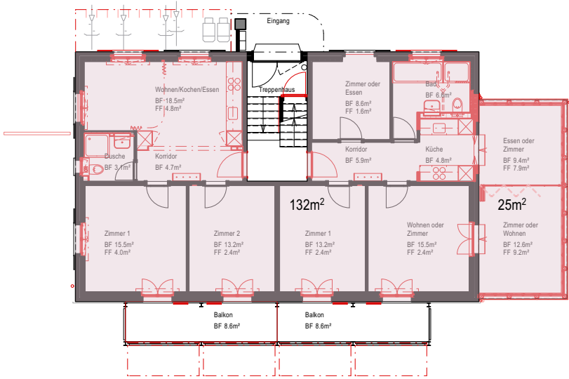
Erdgeschoss
