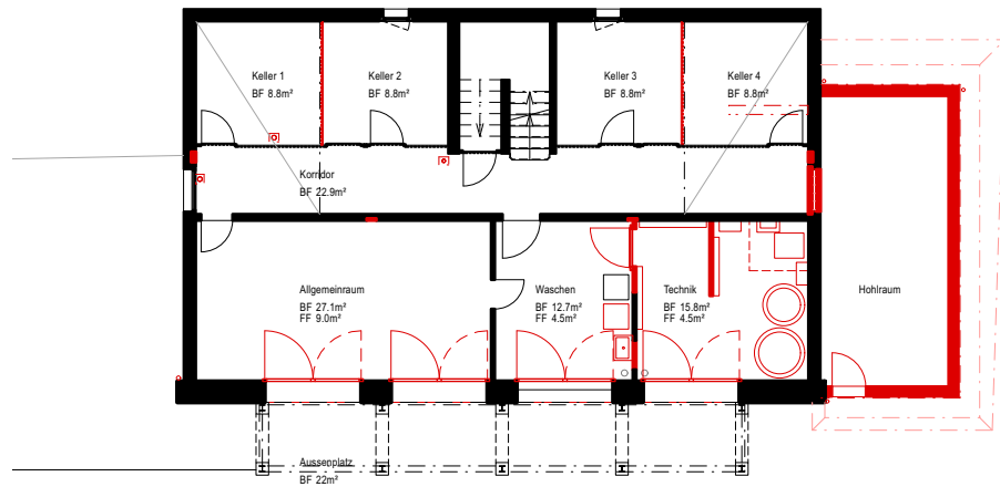
Untergeschoss
