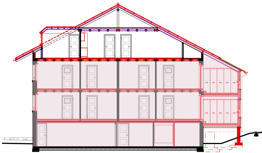
Schnitt B-B
