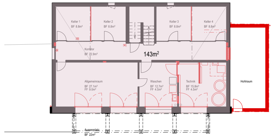
Untergeschoss
