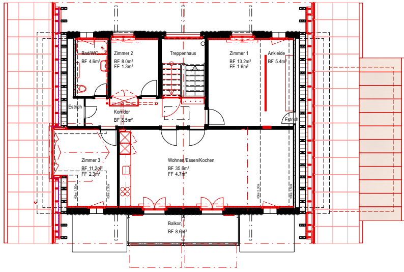
Dachgeschoss
