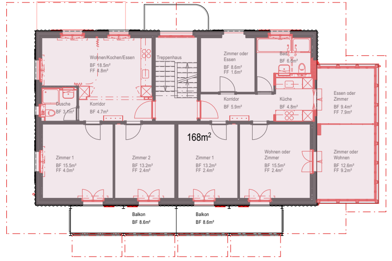
Obergeschoss
