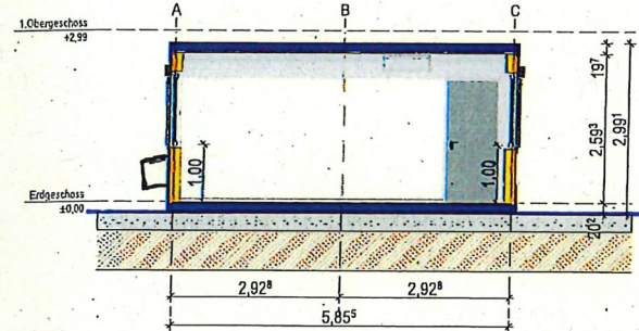
B-B
