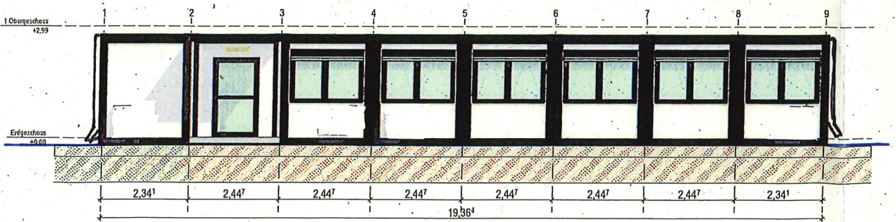
Ansicht C
