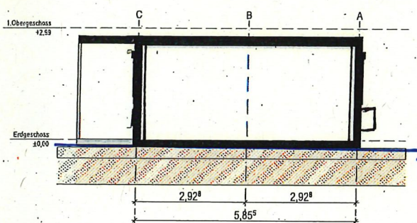
Ansicht B
