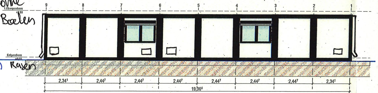
Ansicht A
