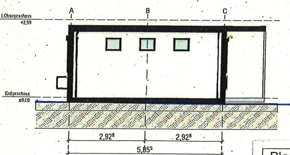
Ansicht D
